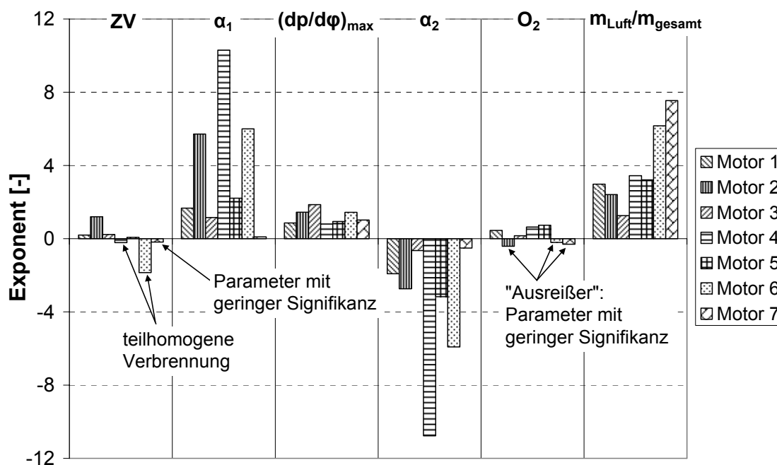
Abb. 6.27: Berechnete Exponenten der Modellparameter für die verschiedenen Motoren für das NO x -Modell, Zahlenwerte aus Tab. 6.7. Am mathematischen Vorzeichen der Exponenten lässt sich die Richtung (Tendenz) des Einflusses der Parameter auf die NO x -Emissionen erkennen und am Zahlenwert die Stärke des Einflusses.
