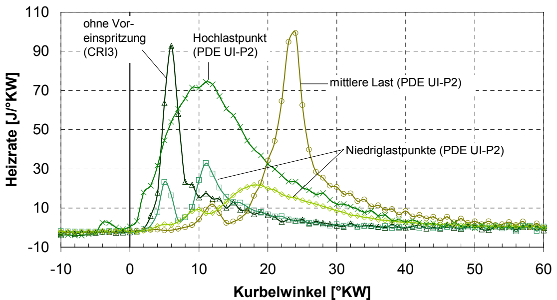
Abb. A. 8: Heizraten bei verschiedenen Betriebszuständen; die Angaben in Klammer beziehen sich auf das verwendete Einspritzsystem; bei der PDE UI-P2 wurde jeweils eine Vor- und eine Haupteinspritzung realisiert
