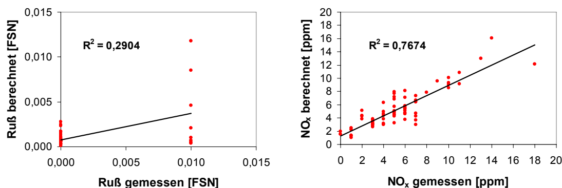
Abb. 7.13: Korrelation zwischen den gemessenen Ruß- und NO x -Emissionen und den mit dem Ruß- bzw. NO x -Modell berechneten Emissionen (homogene Verbrennung bei Verwendung von SuperPlus-Kraftstoff)
