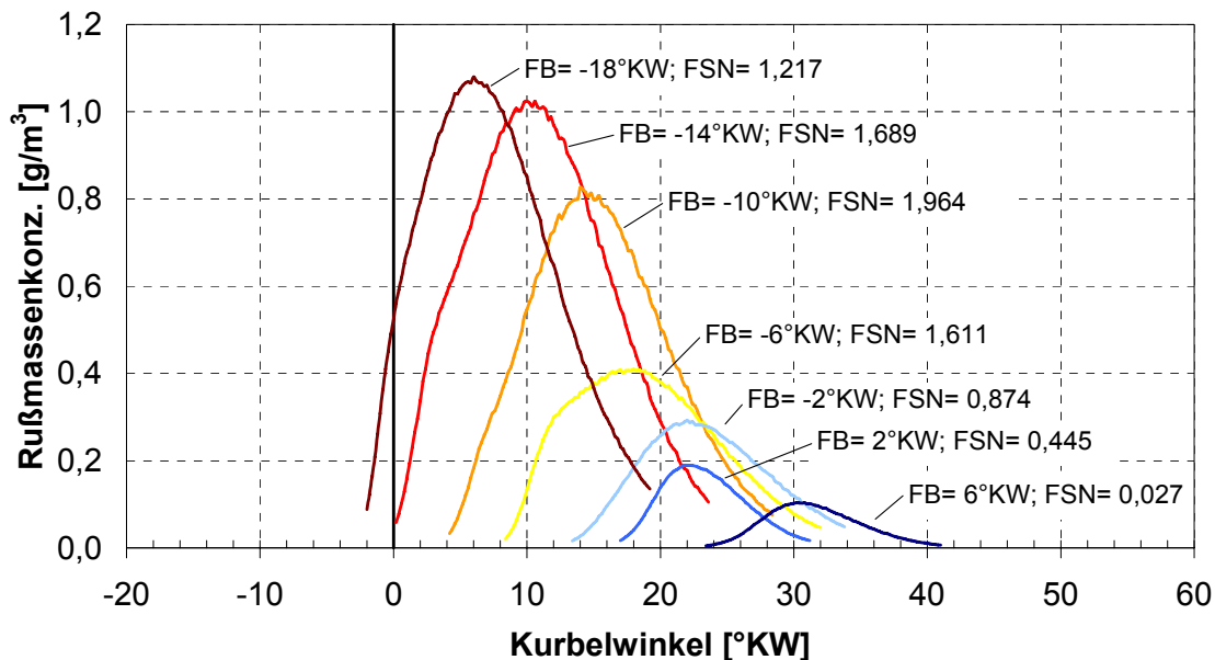
Abb. 6.4: Aus den optischen Messungen berechnete Rußmassenkonzentrationen in [g/m^3] und Angabe der im Abgas gemessenen Rußemissionen in [FSN]^{37} bei einer Förderbeginnvariation bei n = 1400 \text{ U/min} , m_B = 10 \text{ mg/Arbeitsspiel} , AGR = 50 \%
