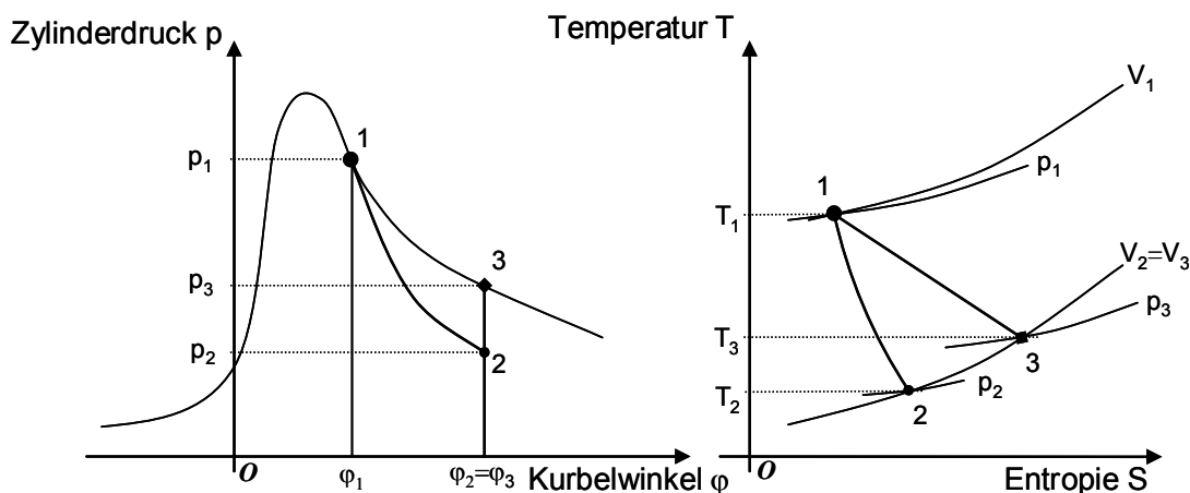
Abb. 4.1: Thermodynamische Zustandsänderungen zur Ermittlung der Heizrate am Beispiel einer Expansion und Wärmezufuhr
