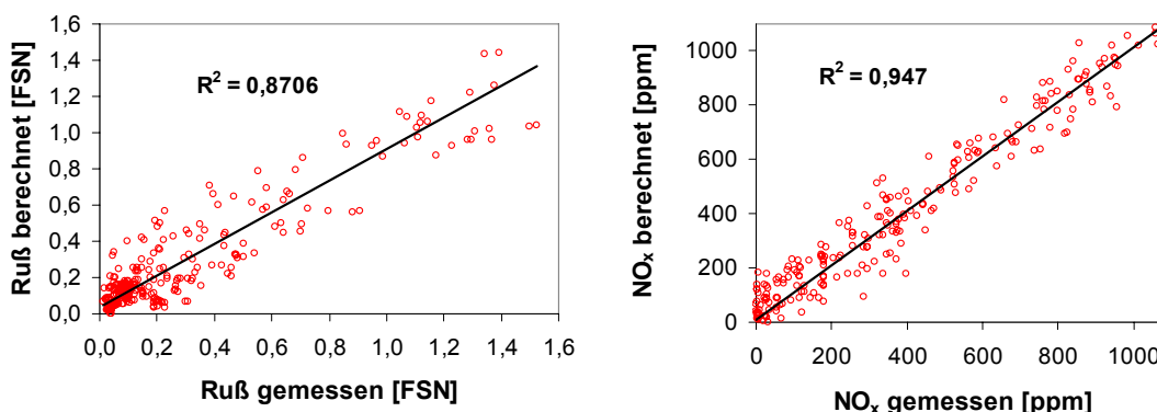
Abb. 6.22: Korrelation zwischen den gemessenen Ruß- und NO x -Emissionen und den mit dem Ruß- bzw. NO x -Modell berechneten Emissionen (FSN begrenzt auf 1,5; NO x begrenzt auf 1100 ppm)
