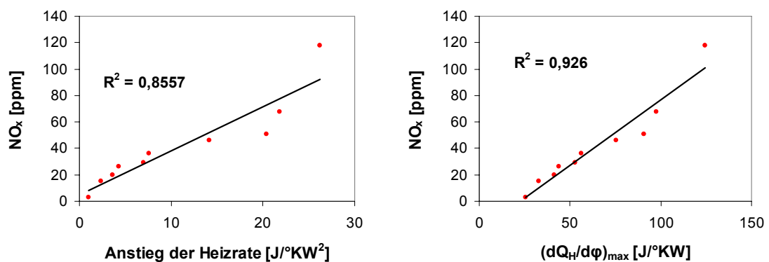
Abb. 6.14: Korrelation zwischen dem Anstieg der Heizrate und den NO x -Emissionen (links) sowie Korrelation zwischen der maximalen Heizrate und den NO x -Emissionen bei einer Förderbeginnvariation von FB = -30^\circ KW bis FB = 6^\circ KW in 4^\circ KW -Schritten bei n = 1400 U/min, m_B = 10 mg/Arbeitsspiel, AGR = 50 %
