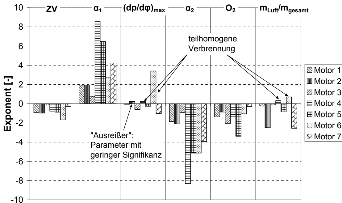
Abb. 6.26: Berechnete Exponenten der Modellparameter für die verschiedenen Motoren für das Rußmodell, Zahlenwerte aus Tab. 6.6. Am mathematischen Vorzeichen der Exponenten lässt sich die Richtung (Tendenz) des Einflusses der Parameter auf die Rußemissionen erkennen und am Zahlenwert die Stärke des Einflusses.
