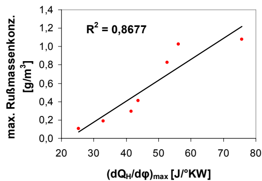
Abb. 6.5: Korrelation zwischen der maximalen Heizrate und der maximalen Rußmassenkonzentration für die oben durchgeführte Förderbeginnvariation bei konstanter Drehzahl, Einspritzmenge und AGR-Rate
