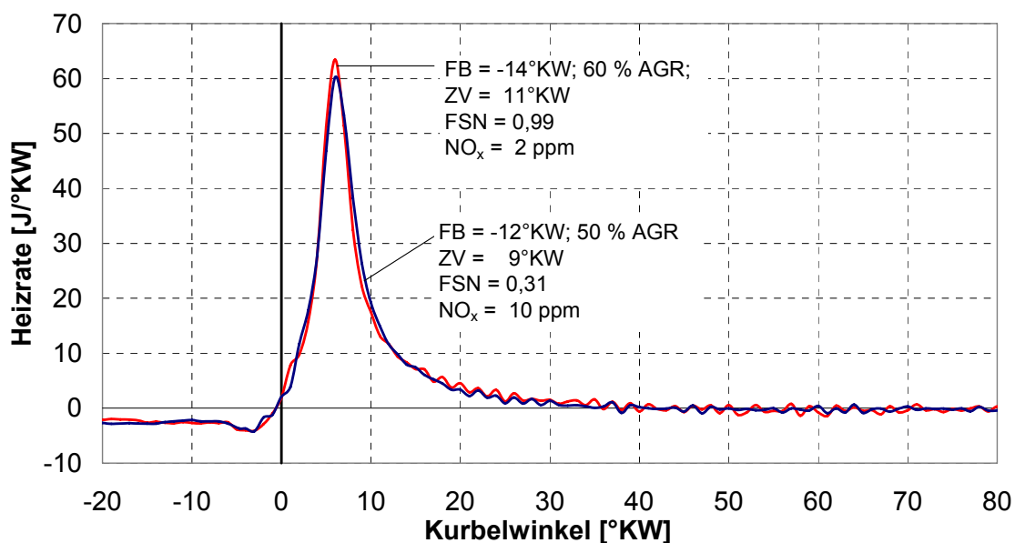
Abb. 6.9: Heizraten bei einer Förderbeginn- und AGR-Variation bei n = 1400 U/min, m_B = 10 mg/Arbeitspiel; im Vergleich zu den anderen hier gezeigten Messungen nur 1 Einspritzung
