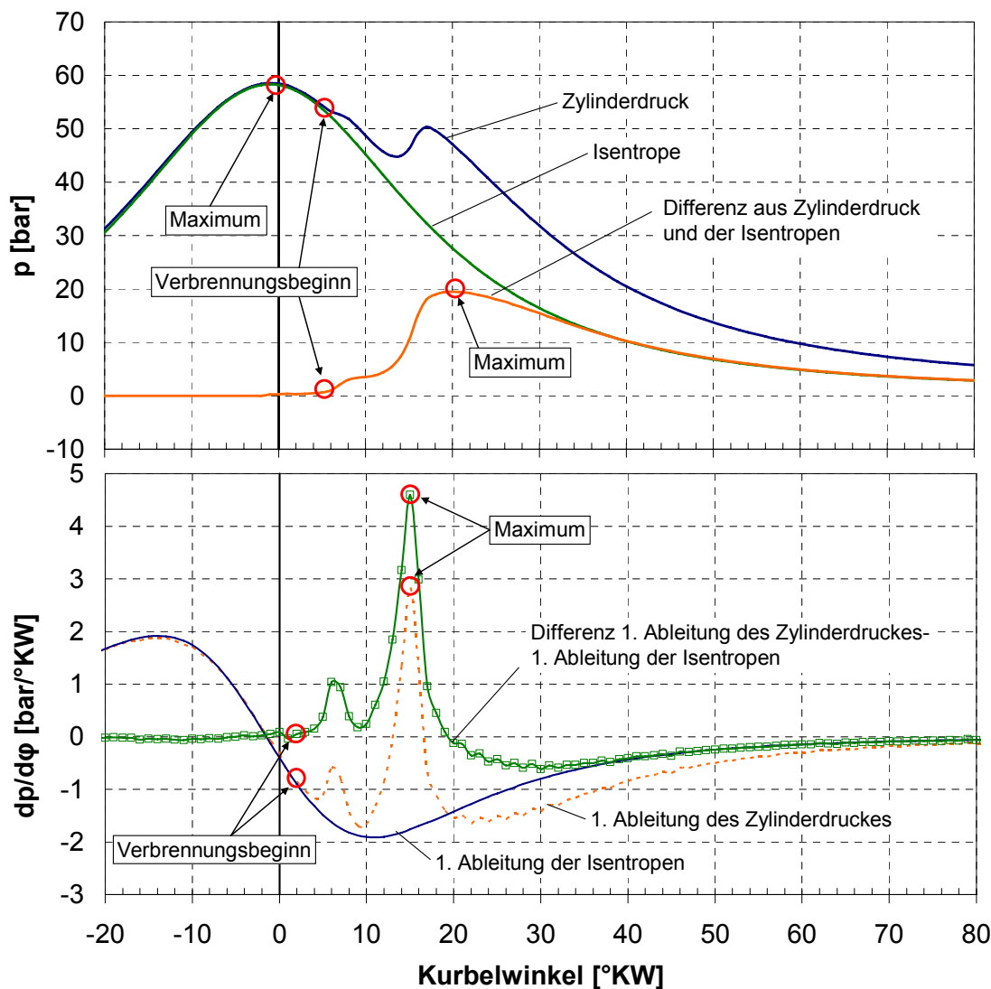
Abb. A. 6: Merkmale aus dem Zylinderdruck (oben) und dessen erster Ableitung
