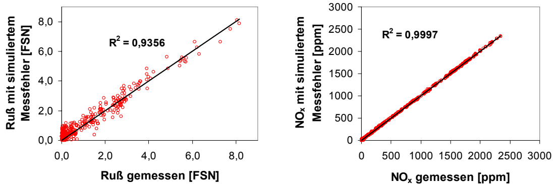
Abb. 6.25: Korrelation zwischen den gemessenen Ruß- und NO x -Emissionen und den nach einer Normalverteilung simulierten fehlerbehafteten Ruß- und NO x -Emissionen
