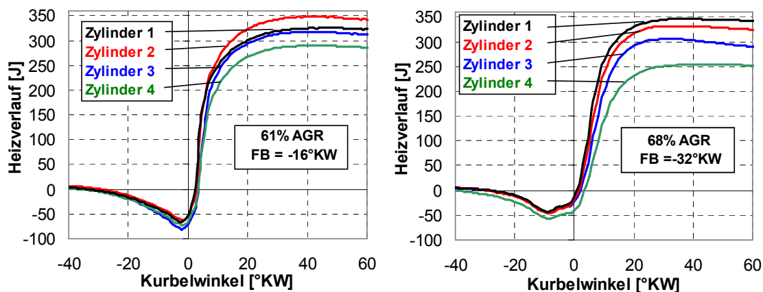
Abb. A. 24: Heizverläufe bei 61 (links) und 68 % AGR in dem Betriebspunkt n = 1400 \text{ U/min} , m_B = 10 \text{ mg/Arbeitsspiel}
