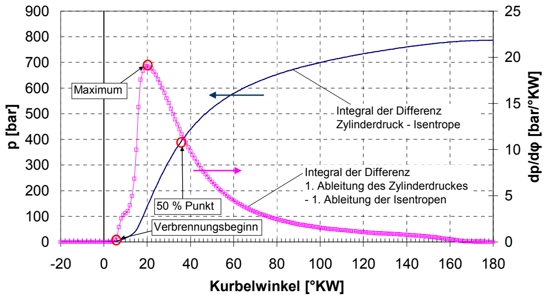
Abb. A. 7: Merkmale aus dem Zylinderdruck und dessen erster Ableitung
