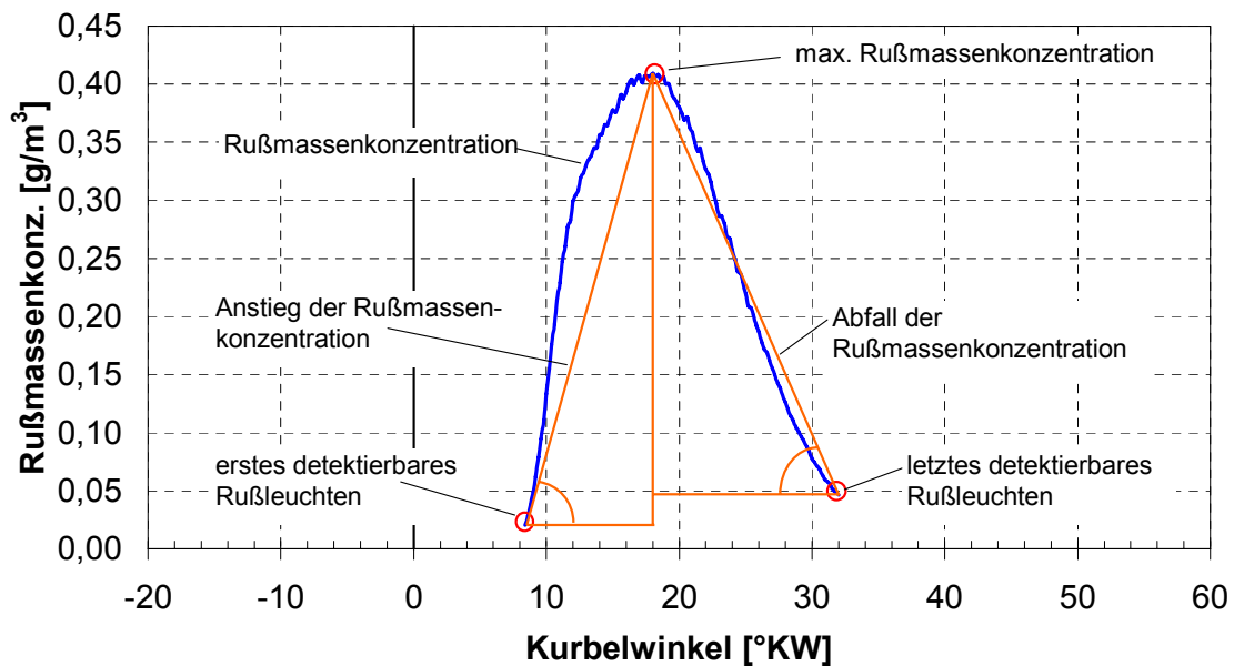
Abb. A. 12: Parameter zur Beschreibung der Rußmassenkonzentration (Prinzipskizze): Anstieg, Maximum und Abfall sowie Hilfsgrößen zu deren Ermittlung
