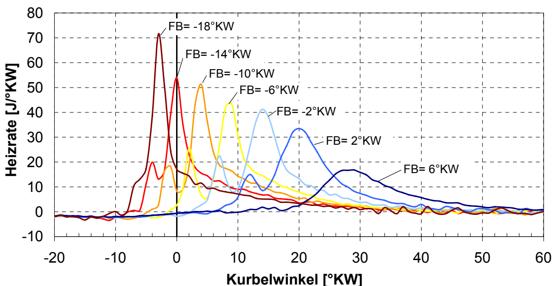
Abb. 6.3: Heizraten bei einer Förderbeginnvariation bei n = 1400 U/min, m_B = 10 mg/Arbeitsspiel, AGR = 50 %
