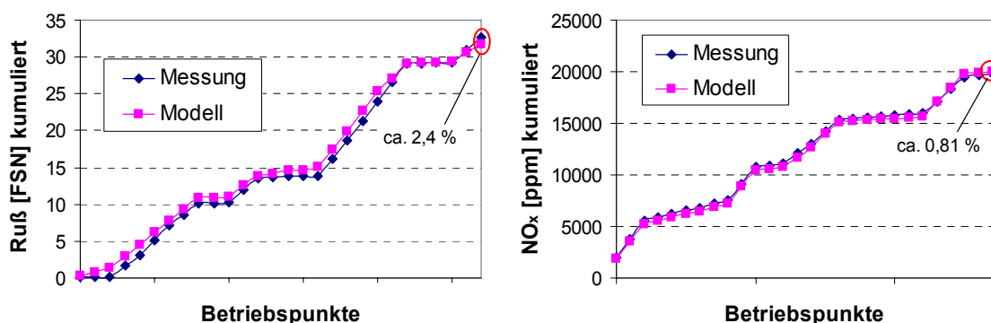
Abb. 6.21: Gemessene und mit dem Ruß- und \text{NO}_x -Modell berechnete kumulierte Emissionen; Angabe von relativer Abweichung zwischen Messung und Rechnung
