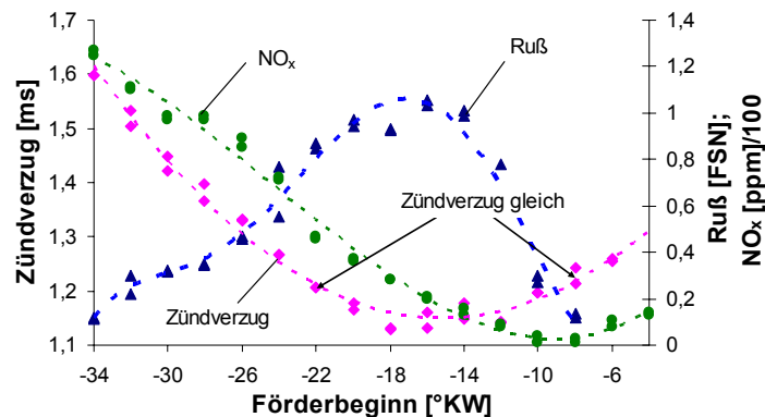
Abb. 7.3: Zündverzug, Ruß- und \text{NO}_x -Emissionen über dem Förderbeginn für den Betriebspunkt n = 1400 \text{ U/min} , m_B = 10 \text{ mg/Arbeitsspiel} , 60 % AGR
