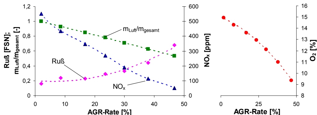
Abb. 7.2: Ruß, \text{NO}_x , m_{\text{Luft}}/m_{\text{gesamt}} und \text{O}_2 über der AGR-Rate bei dem Betriebspunkt n = 1600 \text{ U/min} , p_{\text{mi}} = 3,3 \text{ bar} , \varphi_{\text{QH50\%}} = 5^\circ\text{KW}
