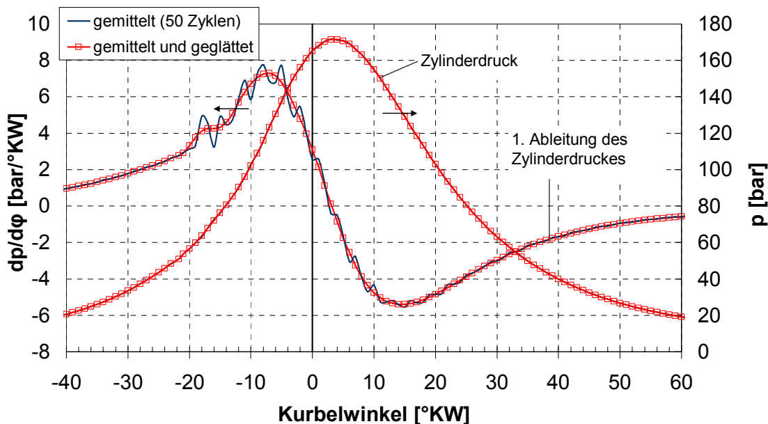
Abb. A. 3: Geglättete und ungeglättete Mittelung des Zylinderdruckverlaufs (nahezu kongruent) und jeweils die daraus berechnete 1. Ableitung in dem Betriebspunkt n = 3500 U/min, FB = -33^\circ KW , 7 % AGR, m_B = 11 mg/Arbeitsspiel
