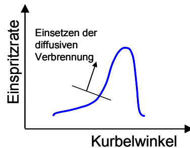
Abb. 7.7: Hypothetische Einspritzverlaufsformung zur Erzielung der „idealen“ Wärmefreisetzung
