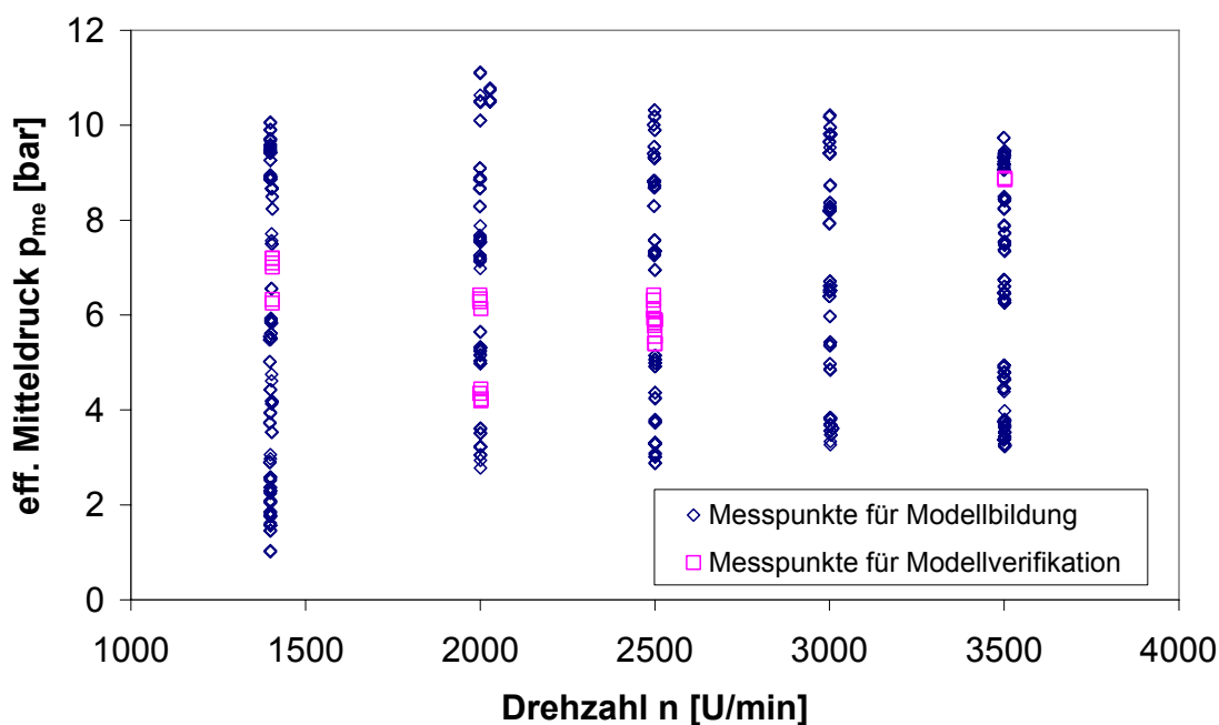
Abb. A. 18: Im Rahmen der Voruntersuchungen vermessener Kennfeldbereich (400 Messpunkte) sowie 28 Messpunkte zur Modellverifikation; den Messpunkten liegt ein D-optimaler Messplan zugrunde
