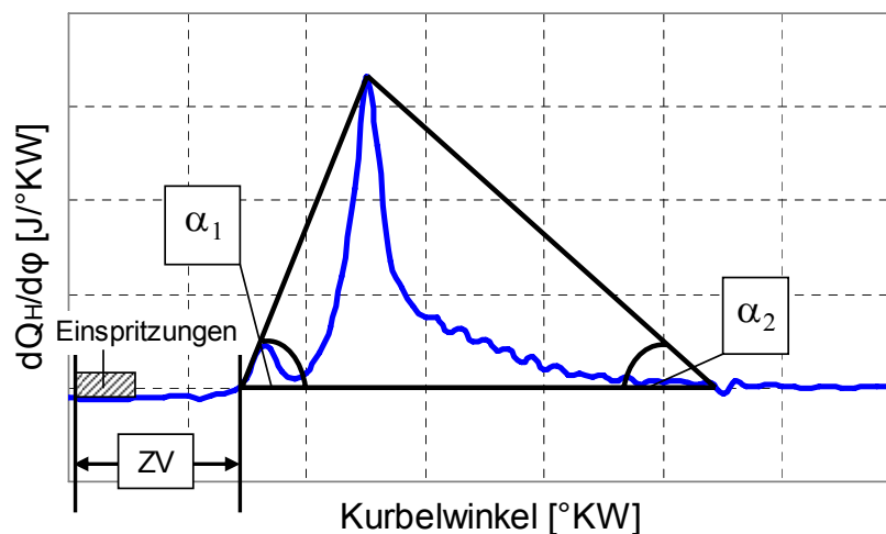
Abb. 6.16: Skizze einer Heizrate mit den ausgewählten Parametern zur Berechnung der Ruß- und \text{NO}_x -Emissionen; mit: ZV – Zündverzug; \alpha_1 – Anstiegswinkel der Heizrate; \alpha_2 – Abfallswinkel der Heizrate; hinzu kommen (nicht in der Abbildung enthalten): (dp/d\phi)_{\text{max}} – maximaler Druckanstieg; O_2 – Sauerstoffkonzentration im Abgas; m_{\text{Luft}}/m_{\text{gesamt}} – Verhältnis der Luftmasse zur Gesamtmasse
