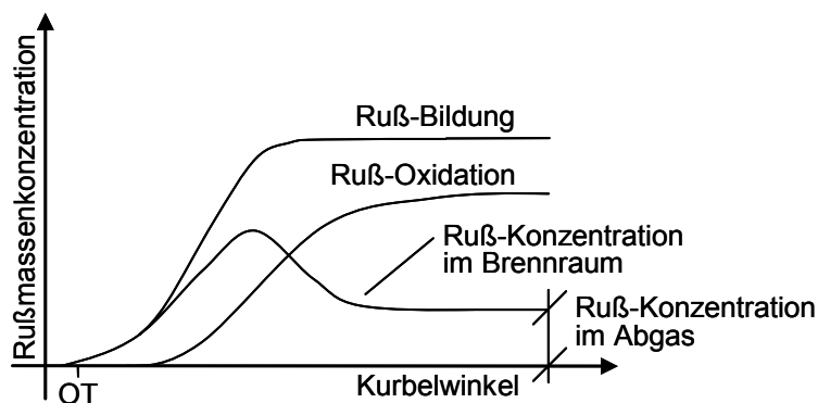
Abb. 6.1: Schematische Darstellung der Verläufe von Rußbildung und -oxidation und der sich daraus ergebenden Rußkonzentration im Brennraum und im Abgas (in Anlehnung an [332])
